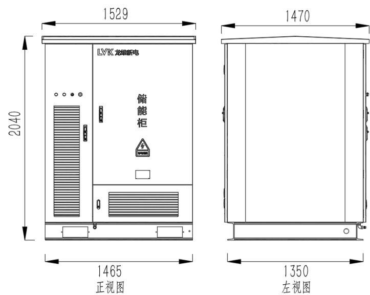
户外柜尺寸图
