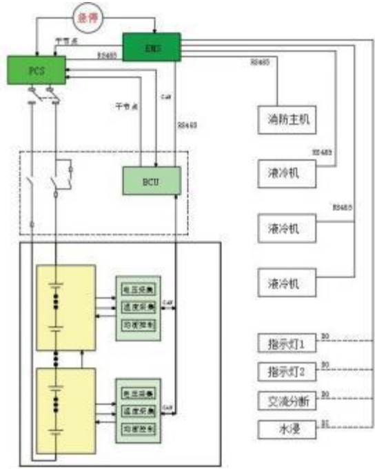
图 2-3 BMS通信架构示意图
